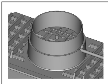
Механизм регулировки тяговой заслонки: закрытое положение
