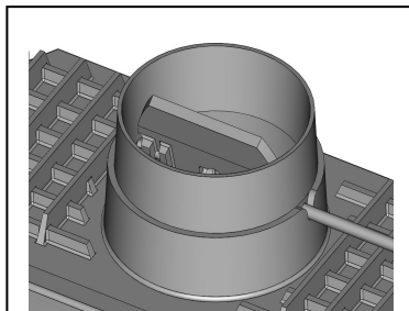
Механизм регулировки тяговой заслонки: открытое положение
