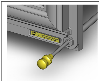
Механизм регулировки тяговой заслонки: открытое положение
