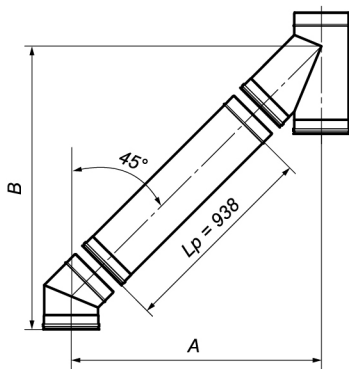
1 отвод 45° + 1 труба L1000 + тройник 45°
