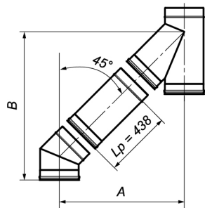
1 отвод 45° + 1 труба L500 + тройник 45°
